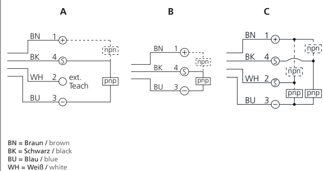
Anschlusschema Connection diagram
