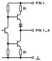
Abb. 3: Transistorausgang
