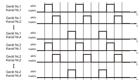
Abb. 4: Funktionsdiagramm Master-Slave-Betrieb
