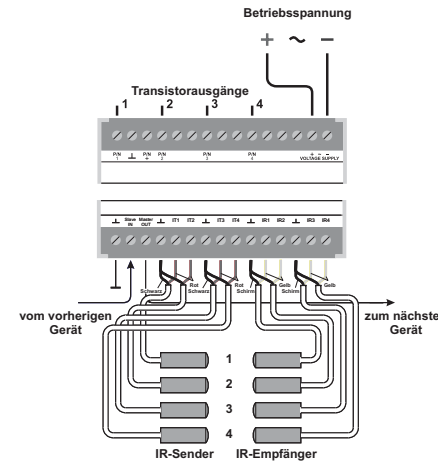
Abb. 2: Anschlussschema
