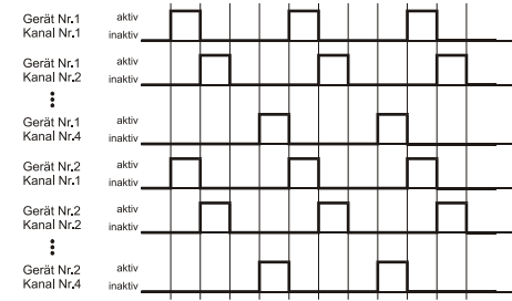
Abb. 4: Funktionsdiagramm Master-Slave-Betrieb
