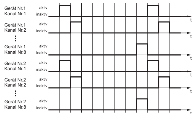
Abb. 4: Funktionsdiagramm Master-Slave-Betrieb
