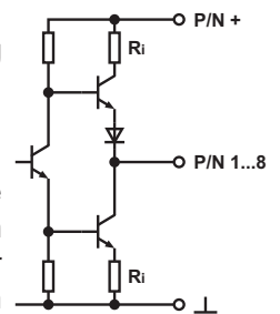
Abb. 3: Transistorausgang
