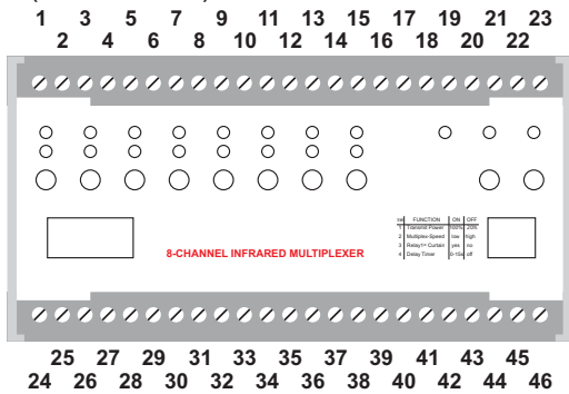
Abb. 1: Klemmen-Nummerierung
