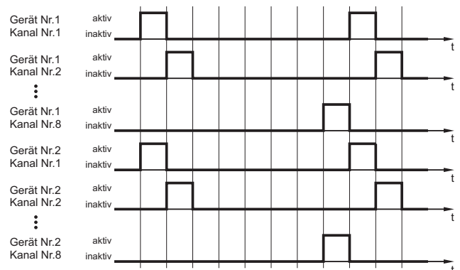
Abb. 4: Funktionsdiagramm Master-Slave-Betrieb
