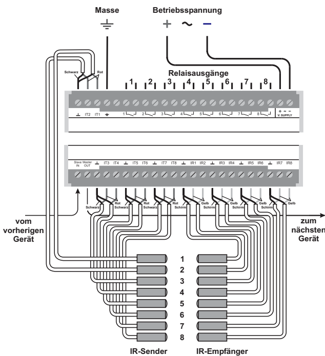
Abb. 2: Anschlussschema
