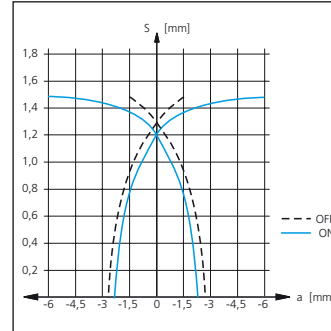
Ansprechkurve M18
